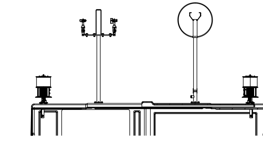
C-C (5:200) Beacon W, rot ES incl. Infrared / Feuer W, rot ES inkl. Infrarot (100 cd)
